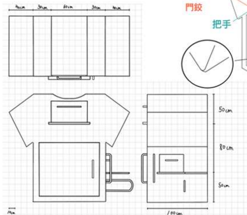
尺寸圖
